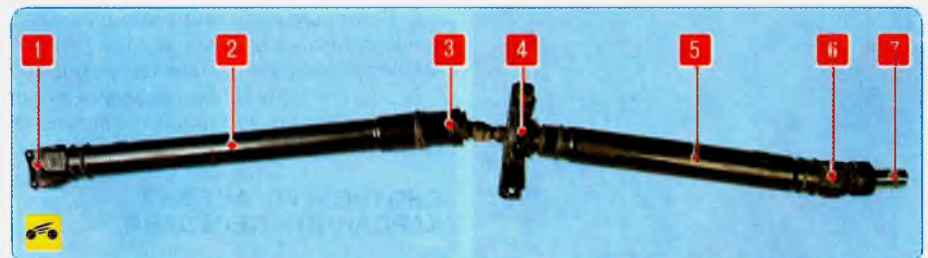
Рис. 6.6. Задняя карданная передача автомобиля с полным приводом: 1 – карданный шарнир заднего вала; 2 – задний вал карданной передачи; 3 – шарнир равных угловых скоростей; 4 – промежуточная опора карданного вала; 5 – передний вал карданной передачи; 6 – карданный шарнир переднего вала; 7 – скользящий шлицевый наконечник вала
